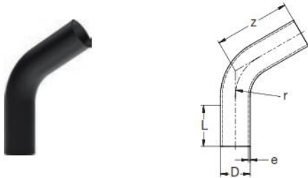
25.60.01.103 PE100 Rohrbogen 60° nahtlos lang SDR11 schwarz PE100 Pipe bend 60° seamless long SDR11 black
