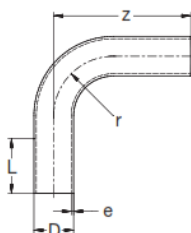
25.90.01.103 PE100 Rohrbogen 90° nahtlos lang SDR11 schwarz PE100 Pipe bend 90° seamless long SDR11 black
