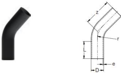
25.45.01.103 PE100 Rohrbogen 45° nahtlos lang SDR11 schwarz PE100 Pipe bend 45° seamless long SDR11 black
