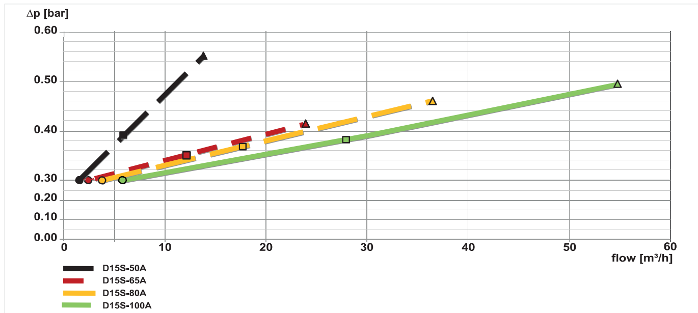
Fig. 2 Perte de charge dans le régulateur en fonction du débit et de la taille de connexion utilisée (DN 50-100) Réglage: P1: 8bar, P2: 3bar
