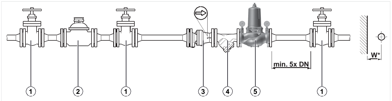
Fig. 1 Exemple d'installation standard
