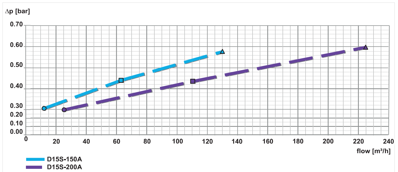
Fig. 3 Perte de charge dans le régulateur en fonction du débit et de la taille de connexion utilisée (DN 150-200) Réglage: P1: 8bar, P2: 3bar
