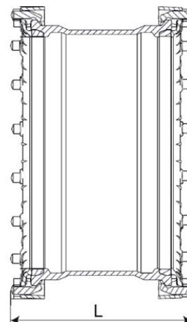
Manchon assemblé avec contrebrides
