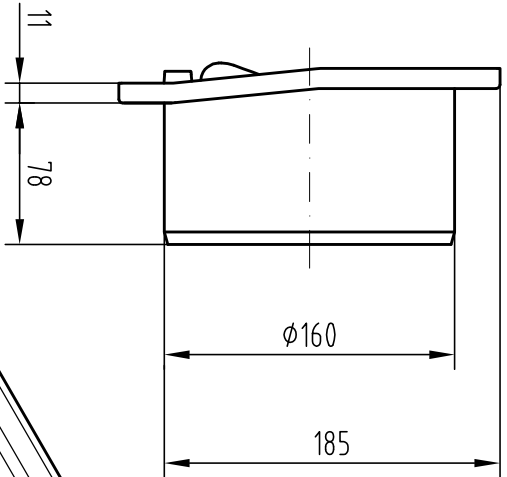
Stirrwand für Rinnenende mit Stützen DN/OD 160 Art.-Nr. 11094
